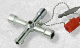
Llave de cabina agua, gas, electricidad WOLFPACK Cod: 02160600
