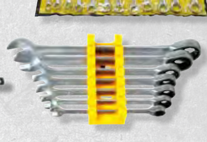
Juego llaves combinada con carraca 7 piezas. Cod: 02326900 MAURER
